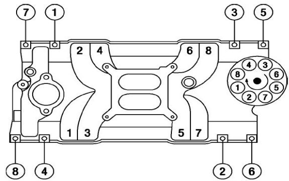
ORDRE D'ALLUMAGE 1-8-4-3-6-5-7-2
