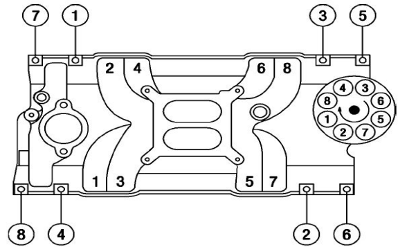
ORDEN DE EXPLOSIÓN 1-8-4-3-6-5-7-2
