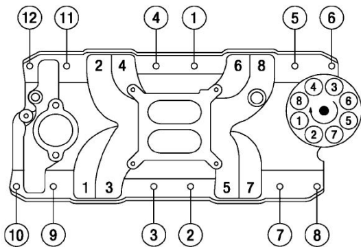
ORDRE D'ALLUMAGE 1-8-4-3-6-5-7-2
