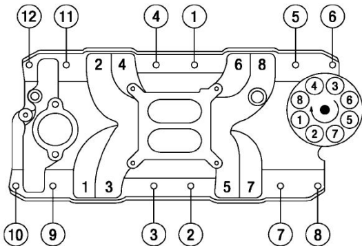
ORDEN DE EXPLOSIÓN 1-8-4-3-6-5-7-2
